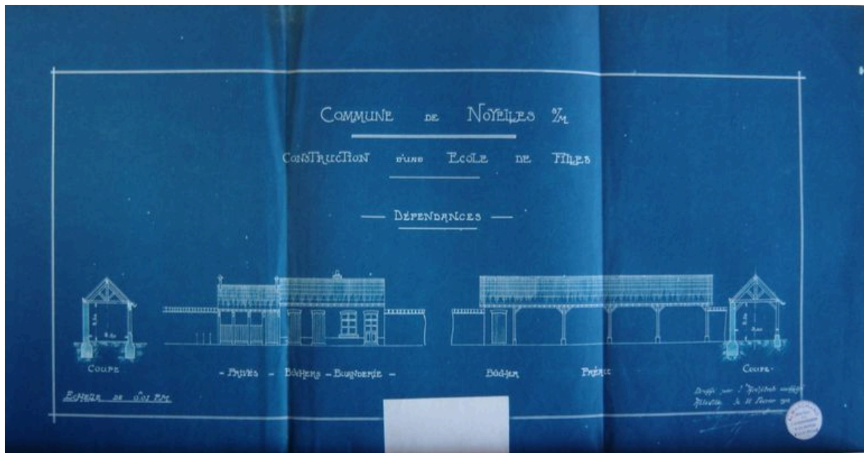
Coupe et élévations des dépendances du projet de la nouvelle école de filles par Alfred Marchand, en 1913.
