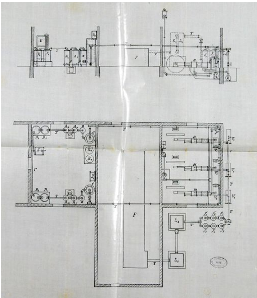
Plan de l'usine Kock, 1899 (AD Oise ; 5Mp2456/1).
