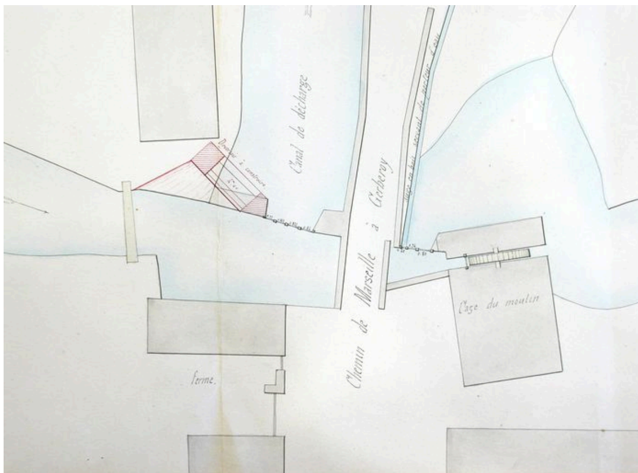
Plan détaillé du moulin de Lachapelle, appartenant à M. de Songeons, 3 août 1852.
