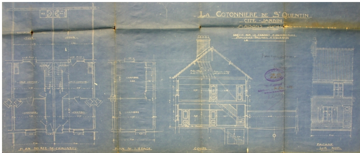
Plans d'une habitation ouvri&egrave;re, par Malgras-Delmas, [1921] (AC Saint-Quentin).
