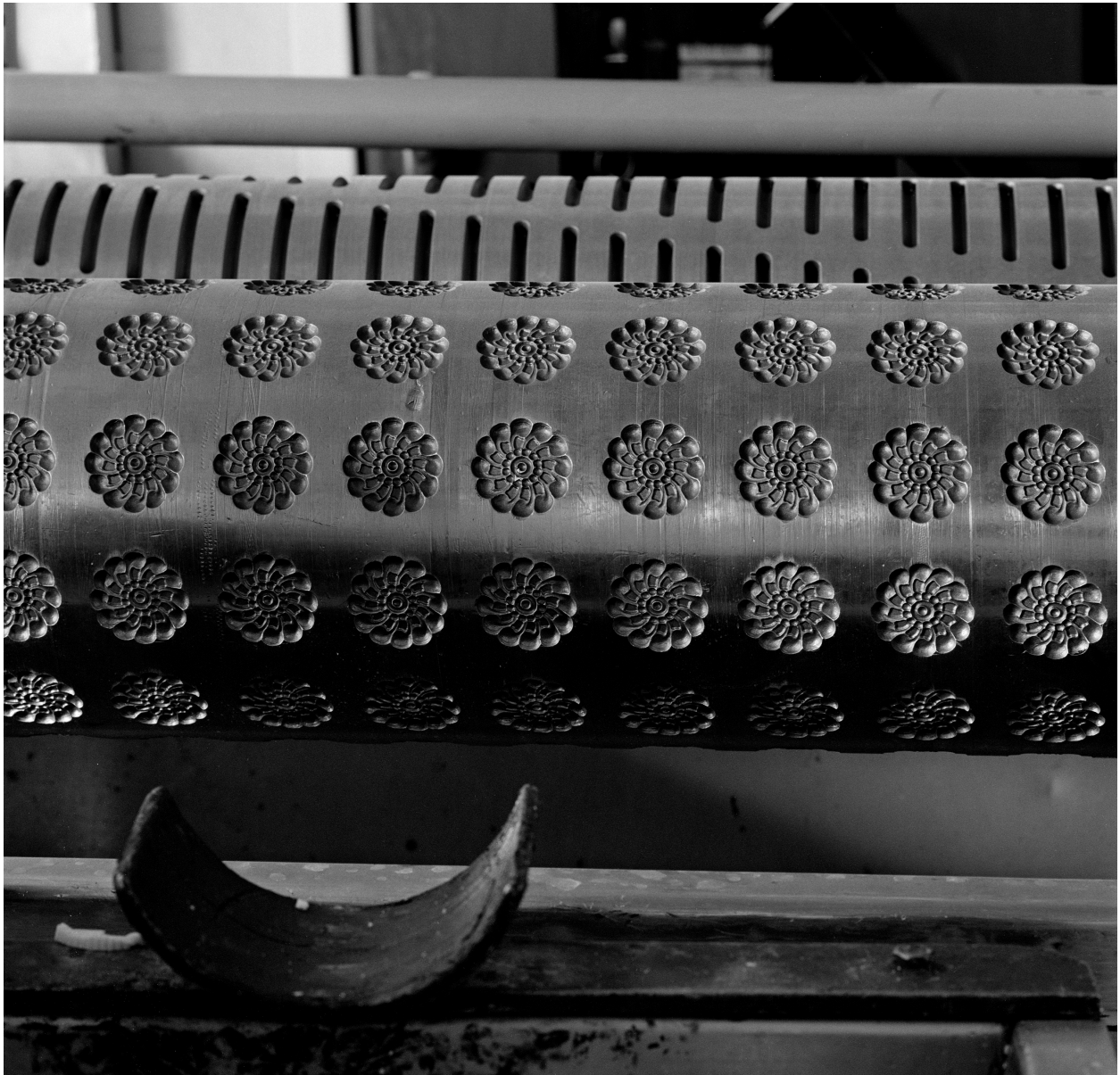
Détail des dessins du cylindre Rota.
