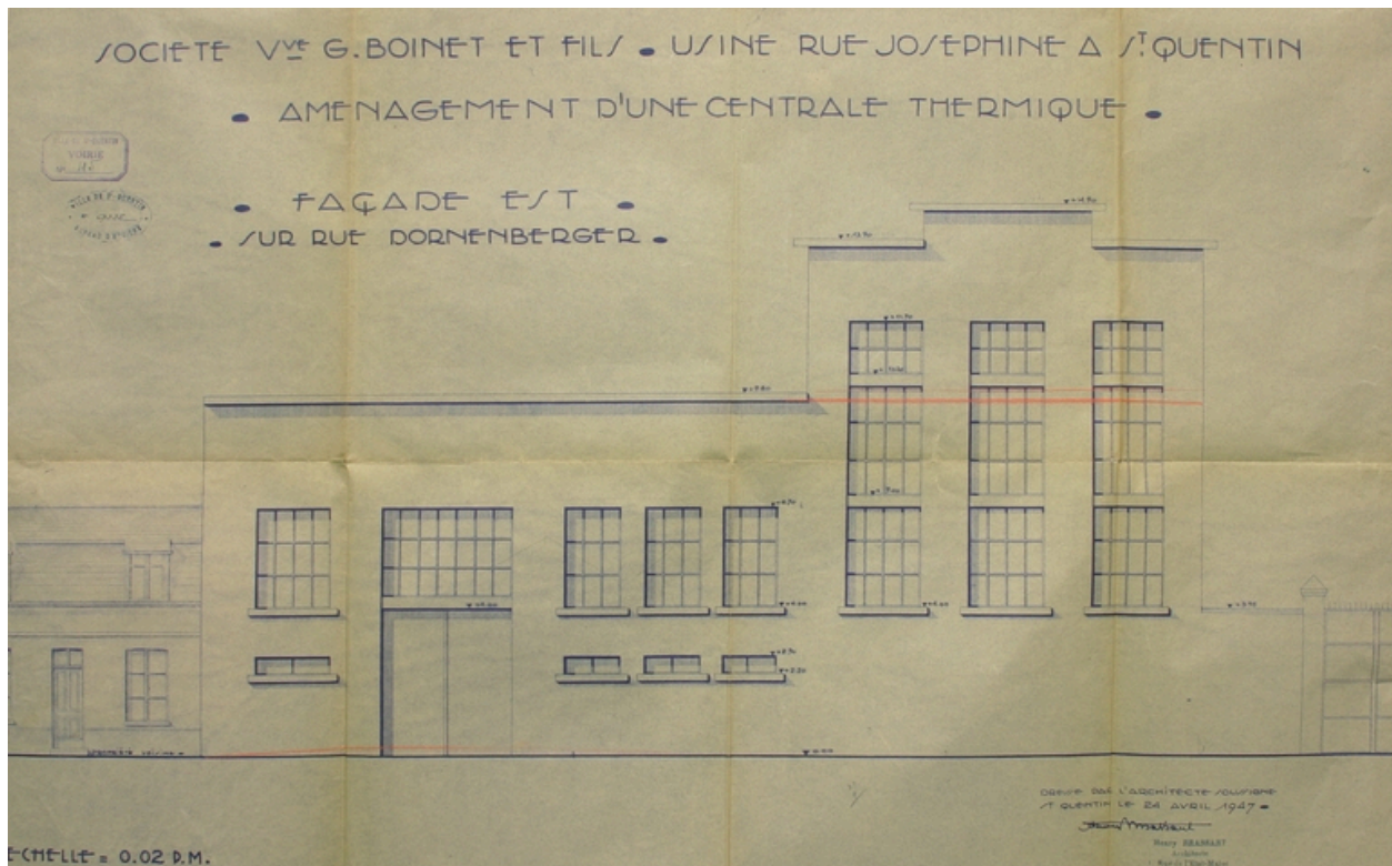
Projet de façade antérieure pour la centrale thermique, par Brassart, 1947 (AC Saint-Quentin).
