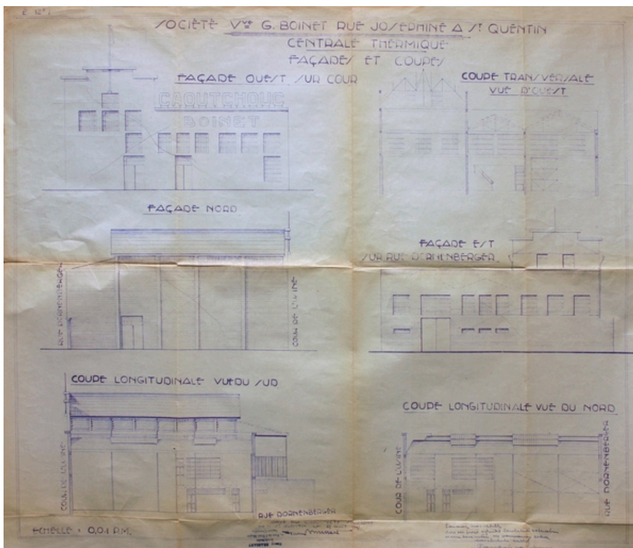
Projet de centrale thermique, par Brassart, 1947 (AC Saint-Quentin).
