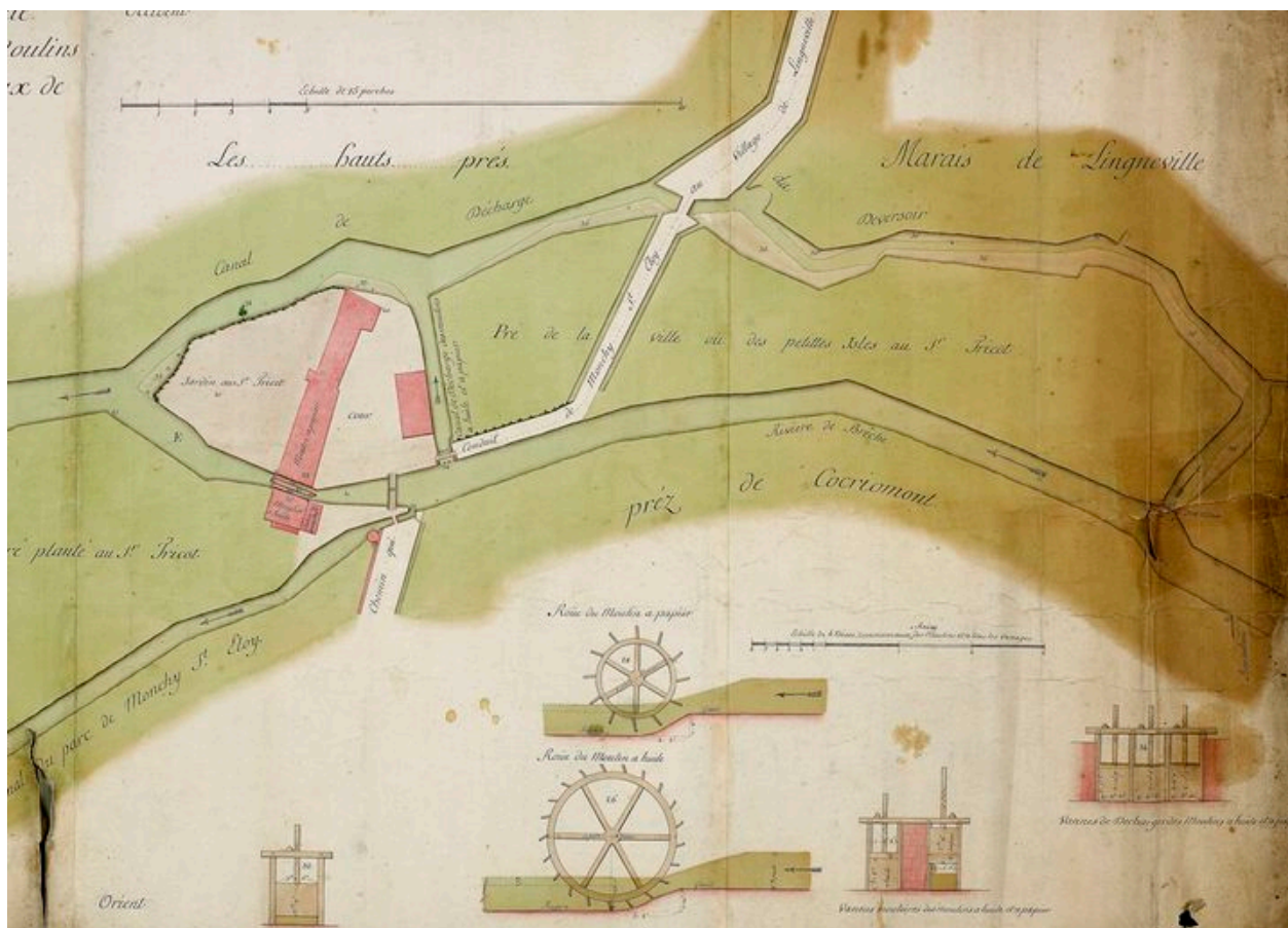
Usine V : Plan du moulin de Caucriamont avant 1793 (AD Oise ; plan 813).
