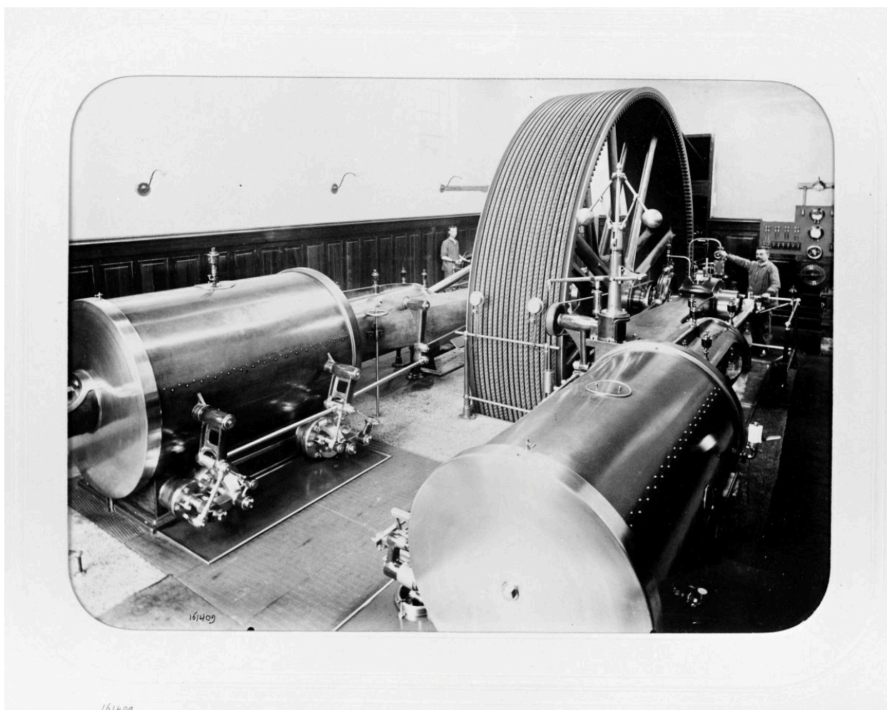
Salle de la machine à vapeur. Photographie de J. David, 1897 (AP Hacot et Colombier).
