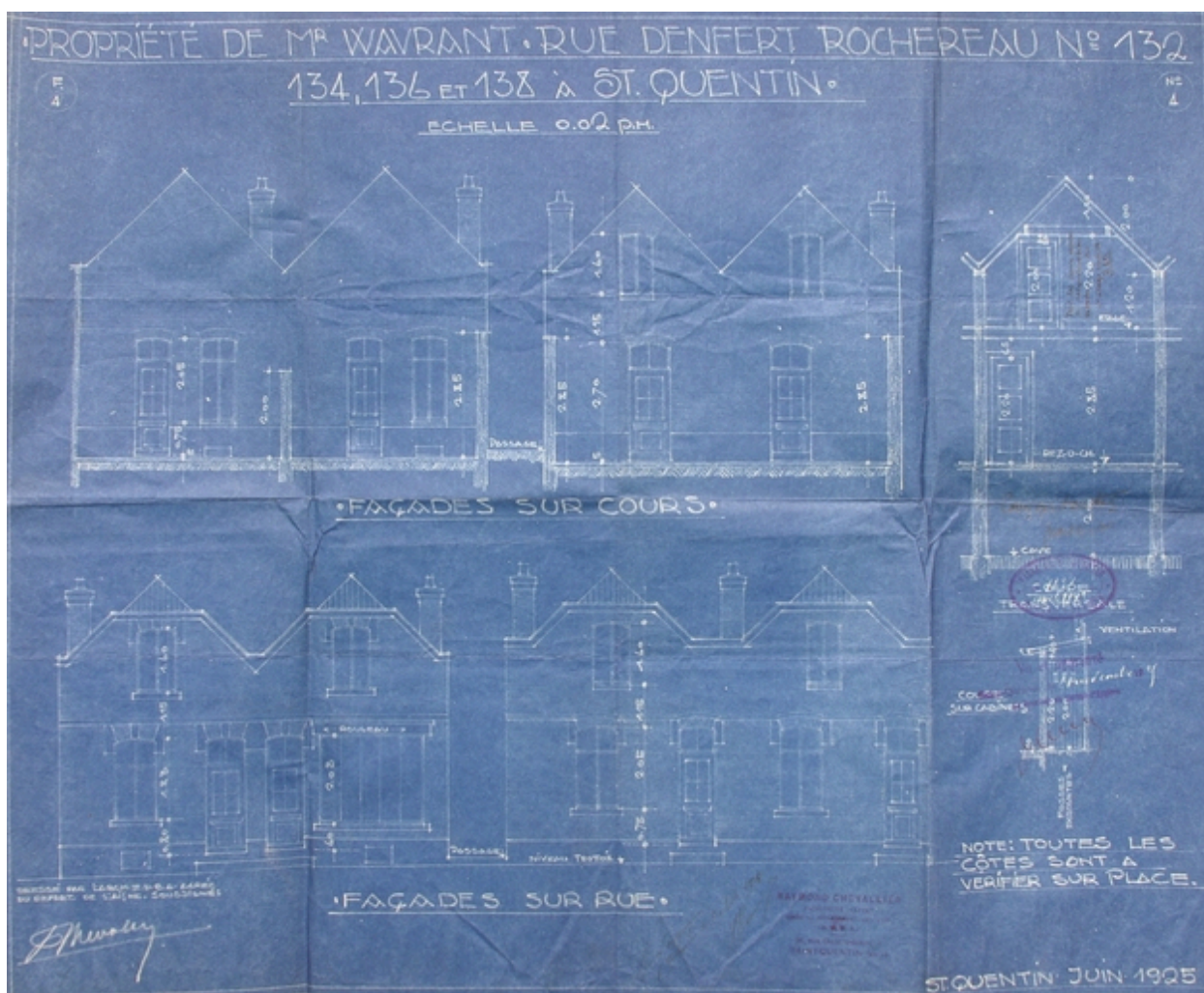
Elévations et coupes des logements sur rue, par R. Chevallier, 1925 (AC Saint-Quentin).
