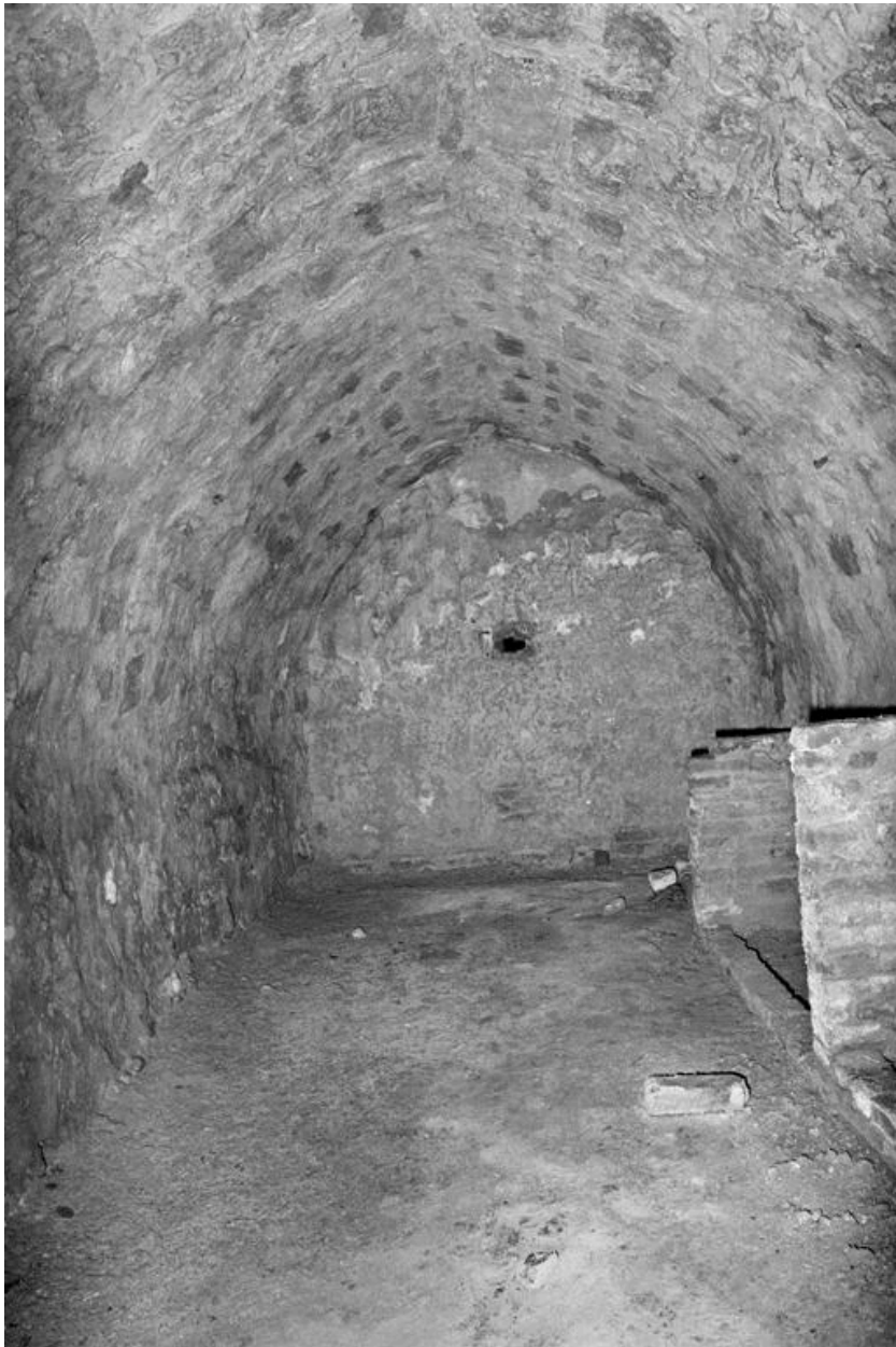
Vue générale du second niveau de cave, couvert d'une voûte en grès en berceau brisé.
