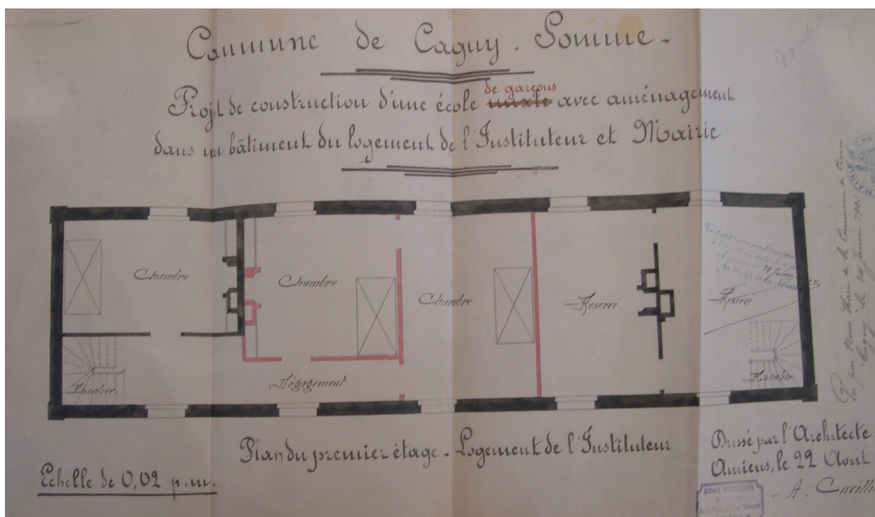
Cagny. Construction d'une école de garçons. Plan de l'étage, dessin, Alfred Cuivillier architecte, 1902 (AD Somme ; 99 O 985).
