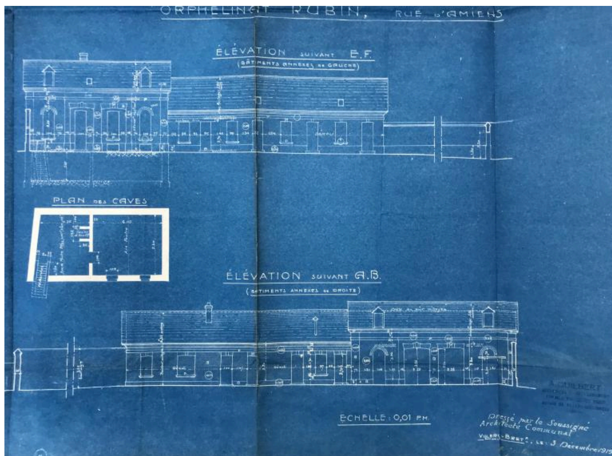
Élévation des bâtiments sur cour. A. Guilbert, 1919 (AD Somme ; 10R 1250).
