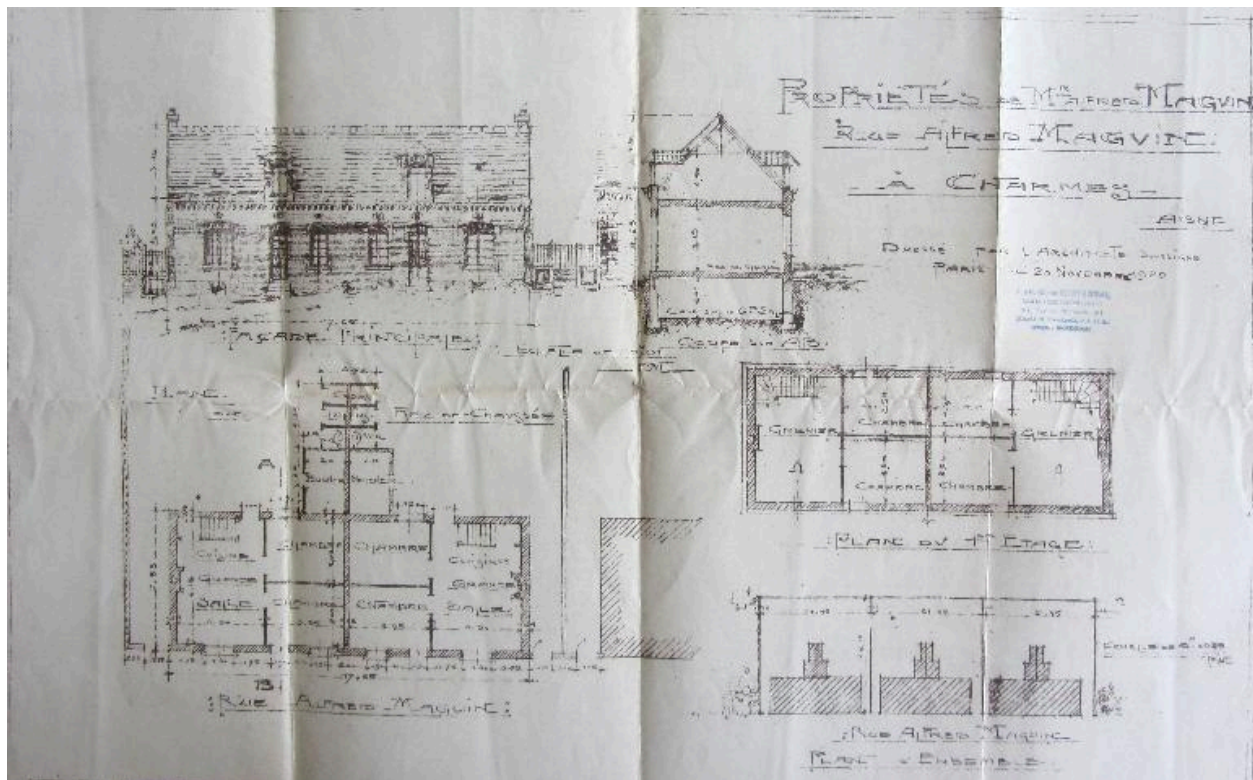
Plans coupes et élévations des trois maisons ouvrières endommagées rue Alfred-Maguin, dressés par J. de Montarnal, 20 novembre 1920 (AD Aisne ; 15 R 772).
