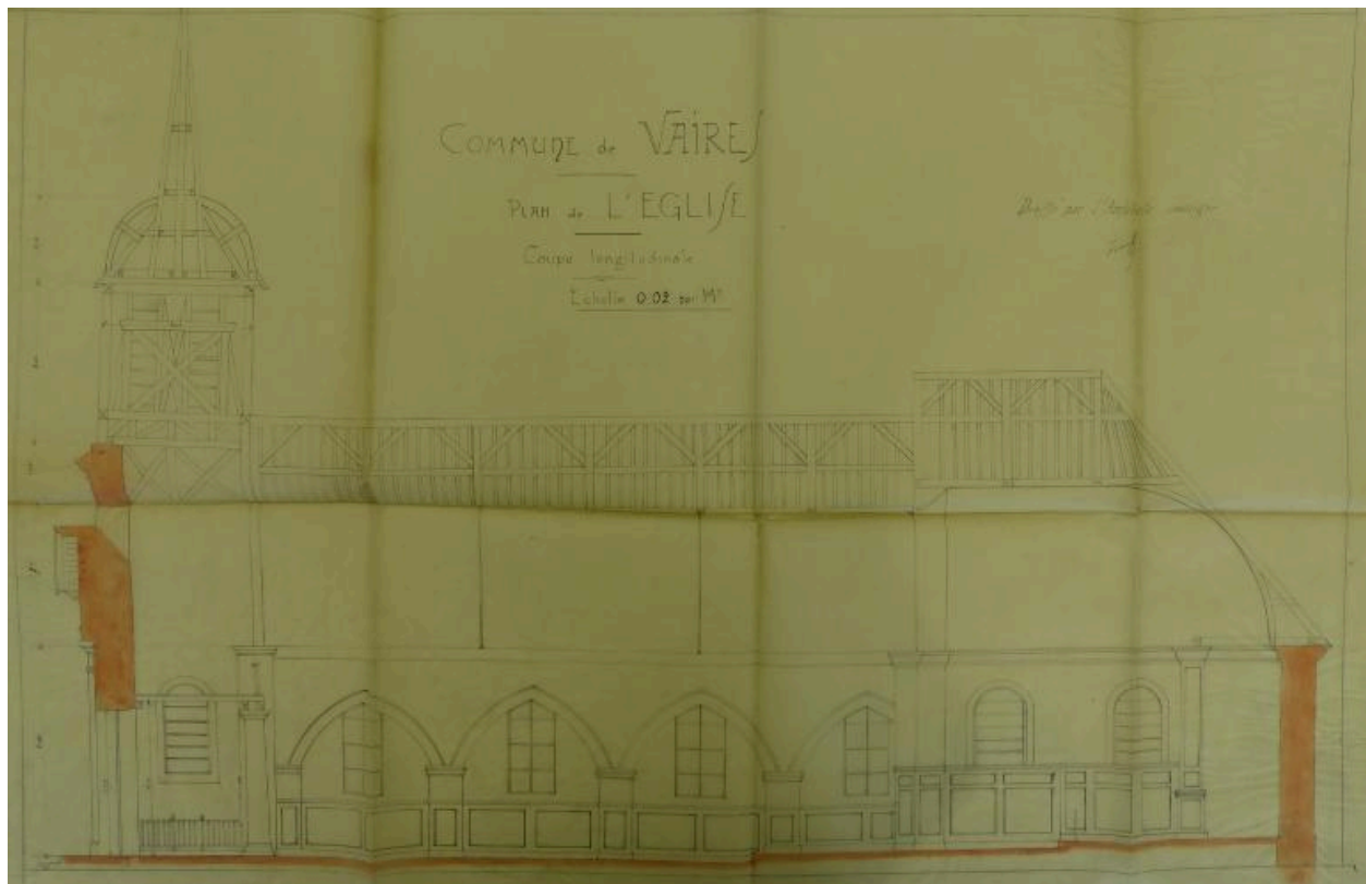
Commune de Vaire-sous-Corbie. L'église. Coupe longitudinale. Relevé effectué pour l'estimation des dommages de guerre, par l'architecte Kueff en 1920 (AD somme ; 10R 1236).
