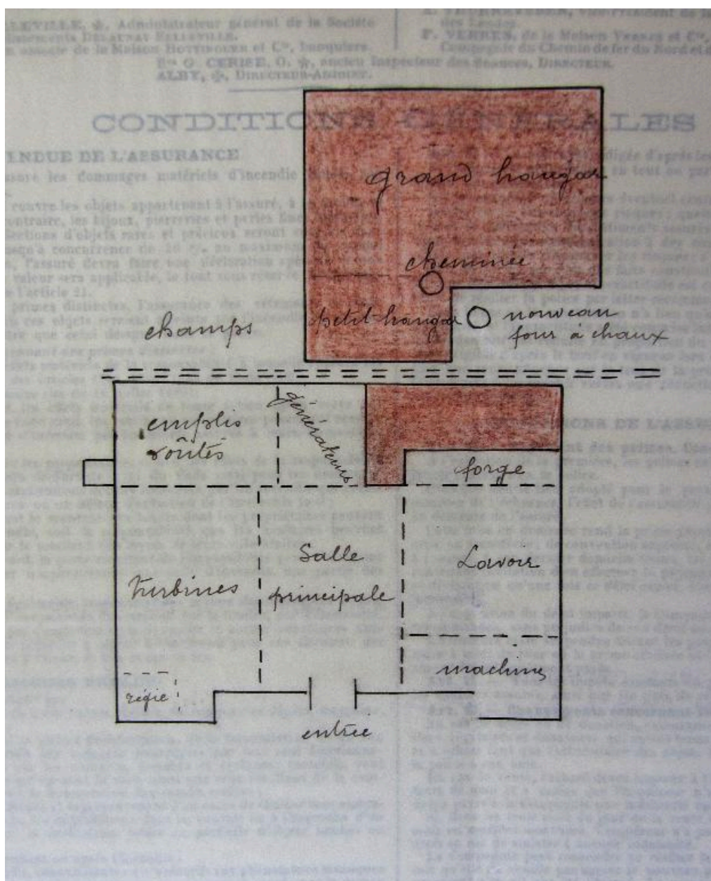
Plan schématique de la sucrerie annexé au contrat d'assurance de l'Union, 1903. (AD Somme ; 10 R 513).
