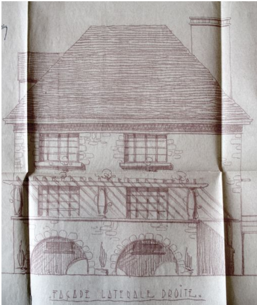
Élévation de la façade latérale droite d'une maison d'ingénieur, par Vally, 1948 (AC Montataire ; 102W1).
