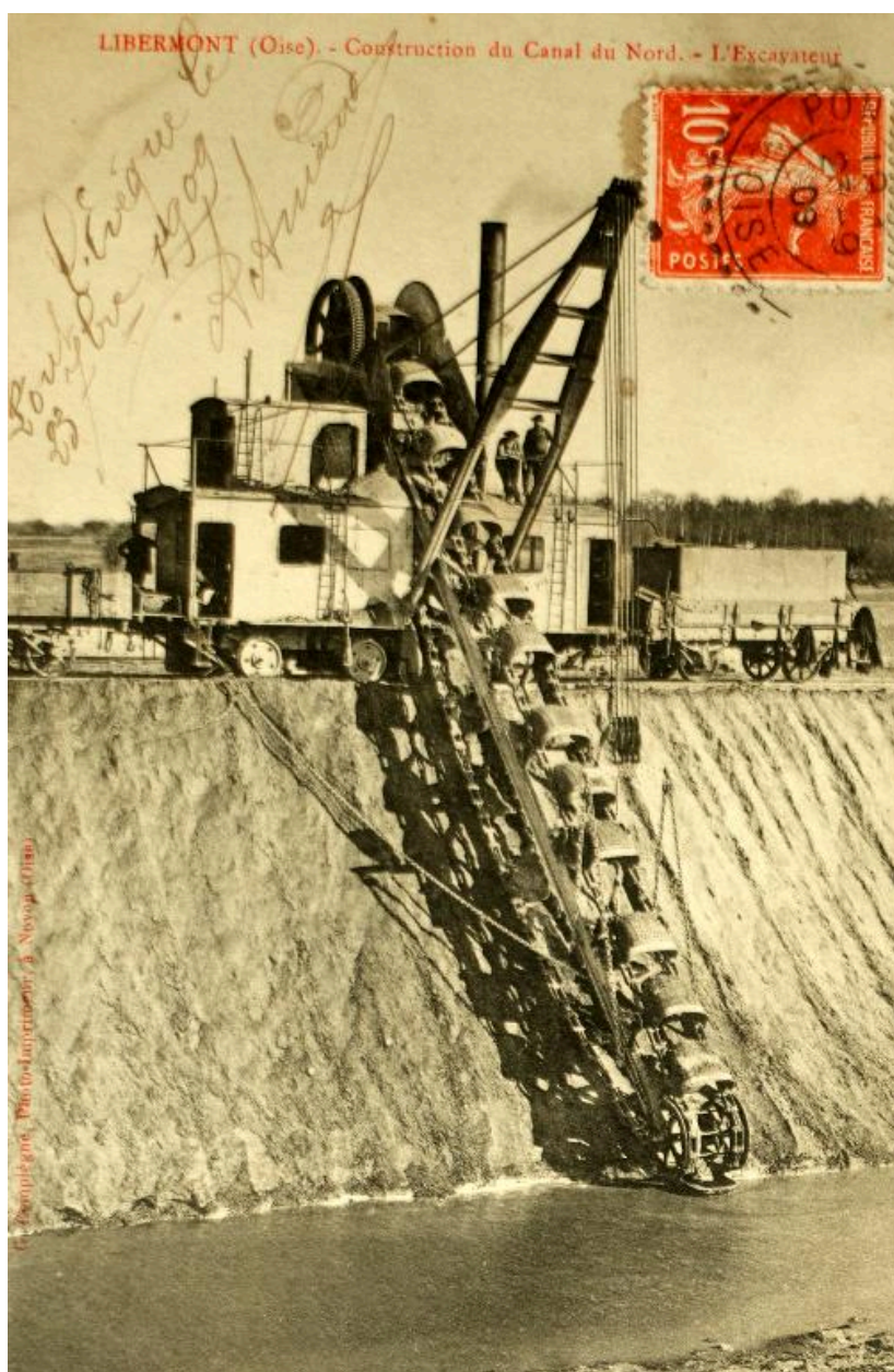
Chantier de construction du canal du Nord. Libermont (Oise), l'excavateur, 1909 (Musée de la batellerie et des voies navigables, Conflans-Sainte-Honorine).
