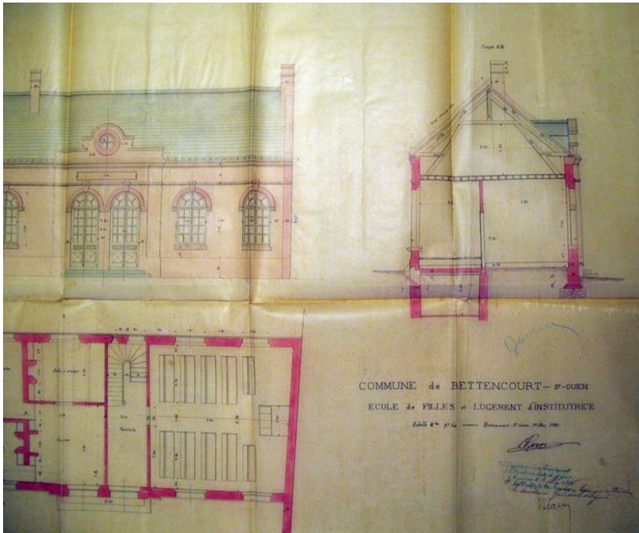
Plan, coupe et façade par Caron, 1894 (AD Somme ; 99 O 710).
