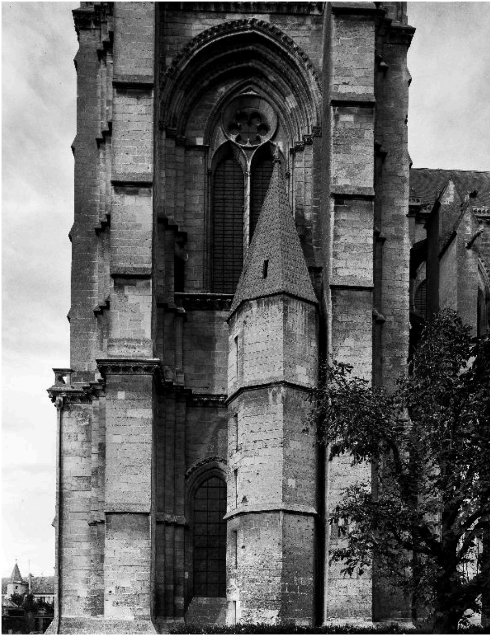
Détail de l'élévation sud de la tour sud-ouest.
