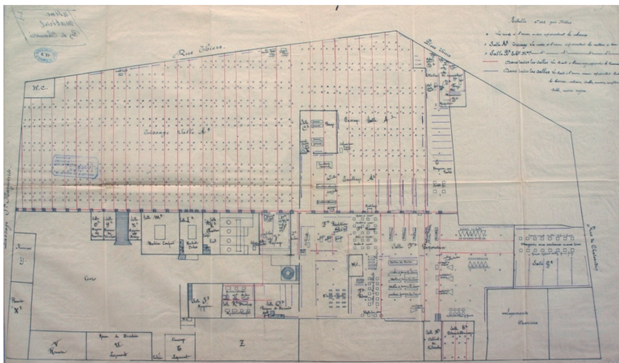
Implantation du matériel au rez-de-chaussée, 1914 (AD Aisne).
