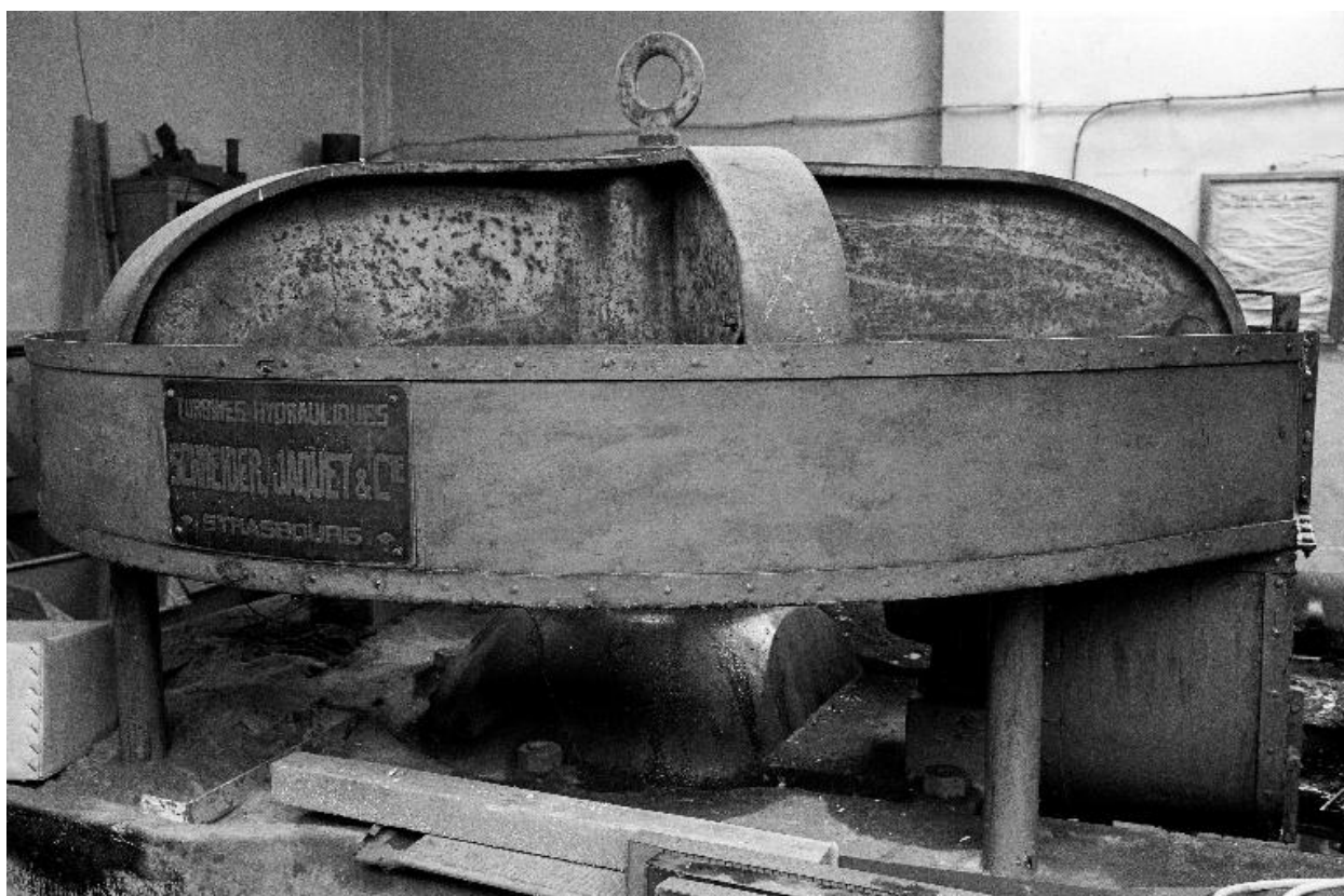
Turbine hydraulique, vue partielle.
