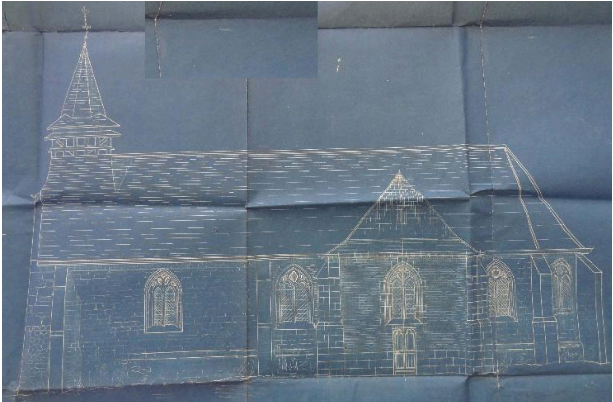
Plan du projet de l'agrandissement de la sacristie : élévation, par Delarue, 1913 (AD Somme ; 99 O 1886).
