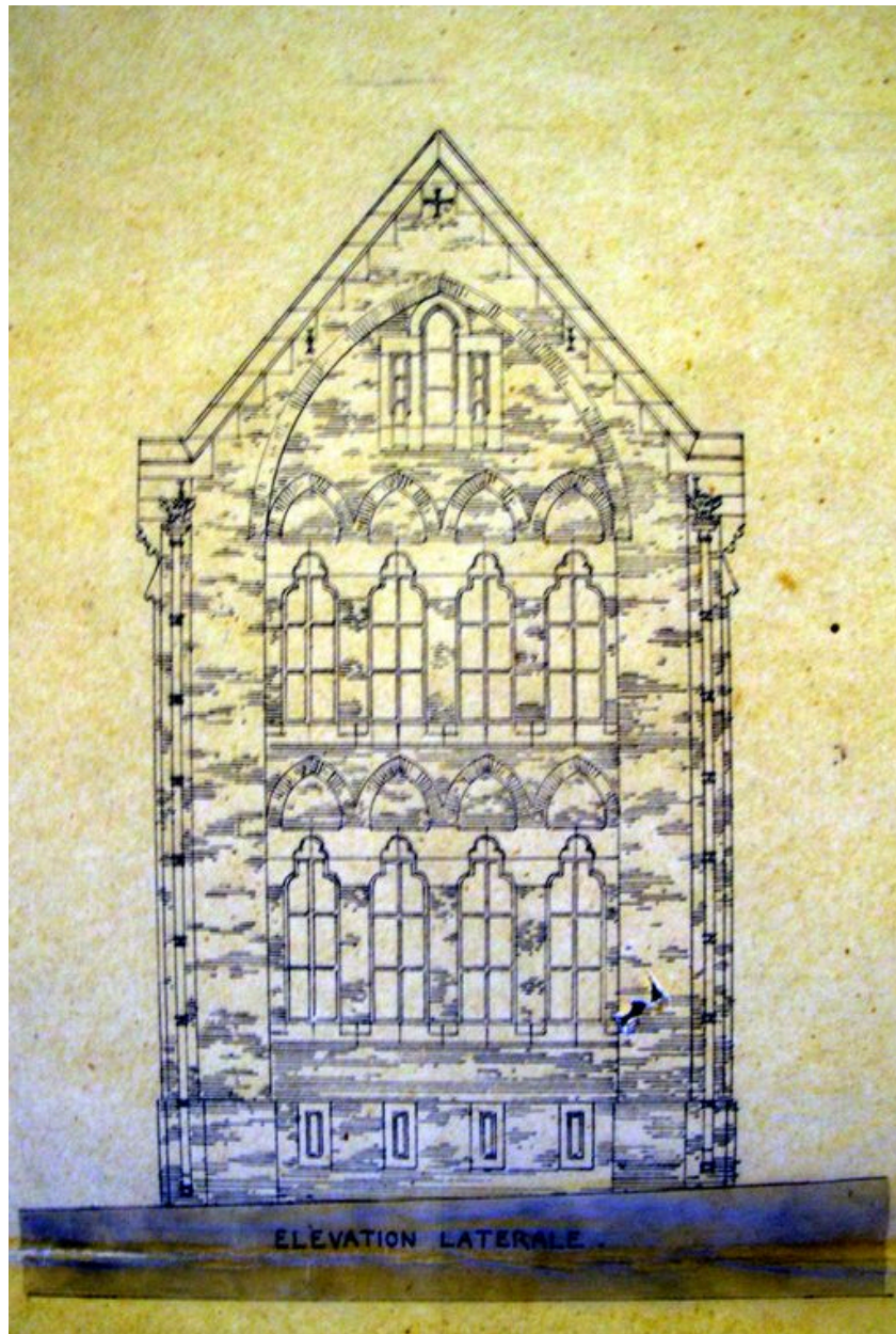
Ecole. Elévation latérale, Massenot architecte, 1856 (AD Somme ; 99 O 1460).
