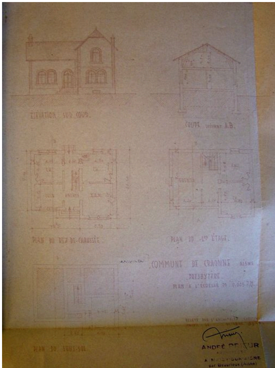
Plan et coupe extraits du dossier de dommages de guerre de la Seconde Guerre mondiale, par André Prieur architecte (AD Aisne : 11 R 8783).
