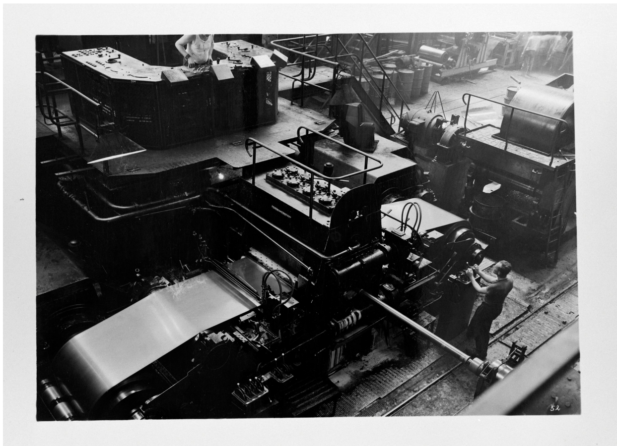
Atelier Rubafer : le laminoir. Photographie ancienne, auteur inconnu, sans date (coll. part.).
