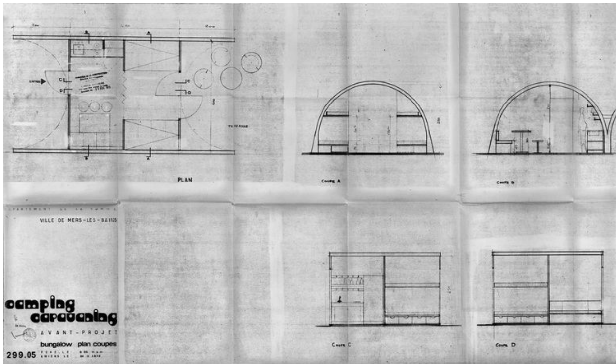
Plans types d'un bungalow (AC Mers-les-Bains).
