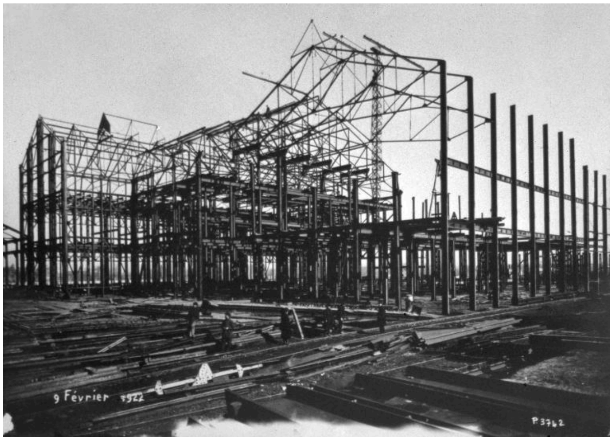
Structure métallique du grand atelier de fabrication de la sucrierie, 9 février 1922 (Archives privées de l'entreprise).
