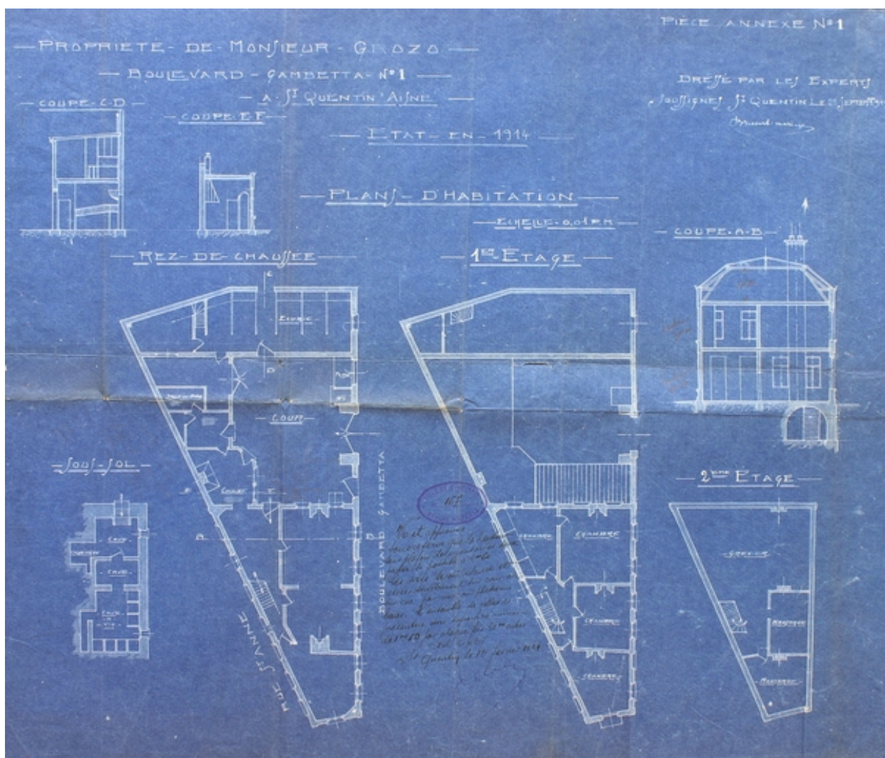
Plan du logement patronal, par Brassart-Mariage, 1914 (AC Saint-Quentin).
