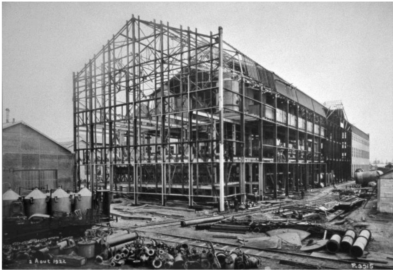
Structure métallique du grand atelier de fabrication, 2 août 1922 (Archives privées de l'entreprise).
