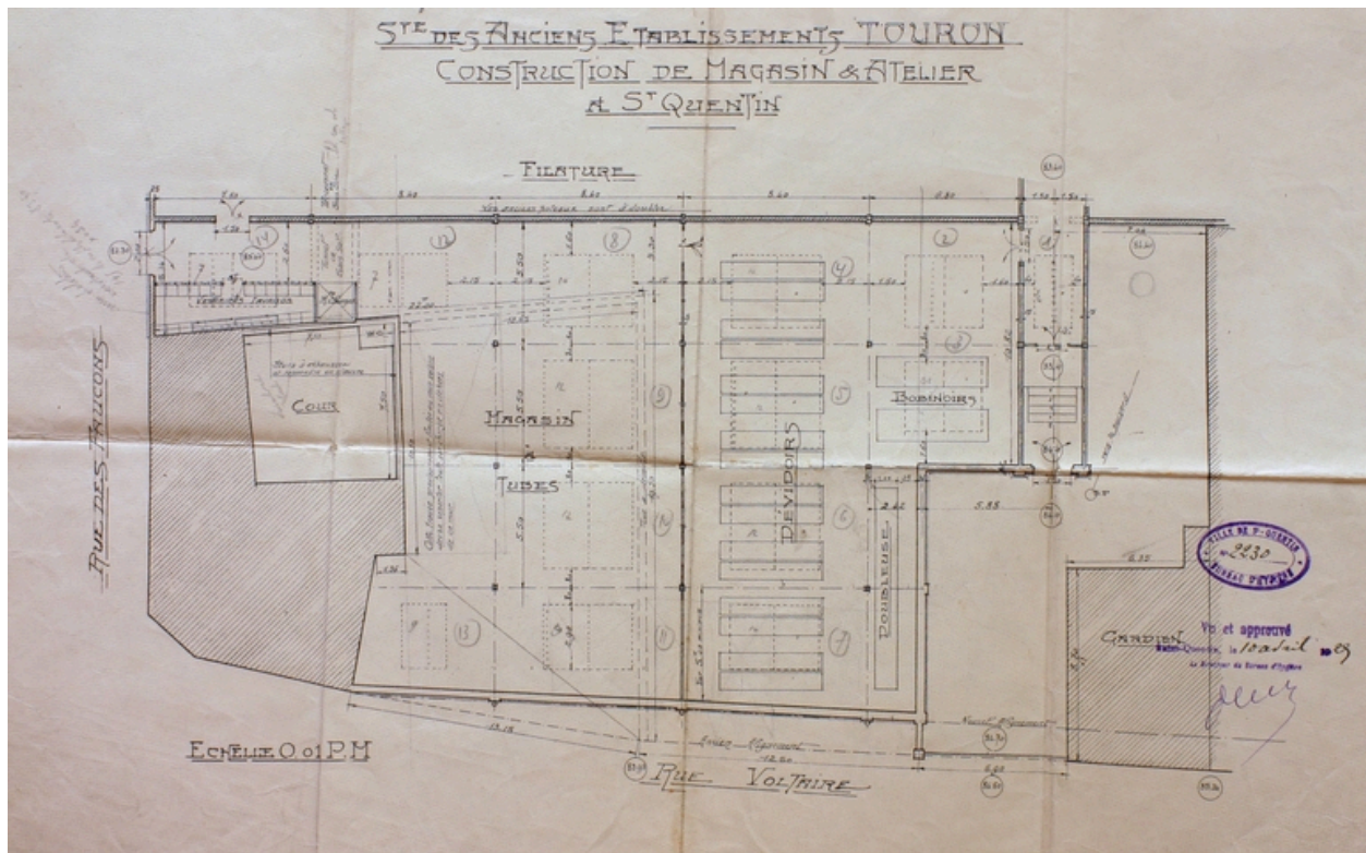
Projet de construction de magasins et ateliers à l'entrée du site, rue Voltaire, par Nalet, 1925 (AC Saint-Quentin).
