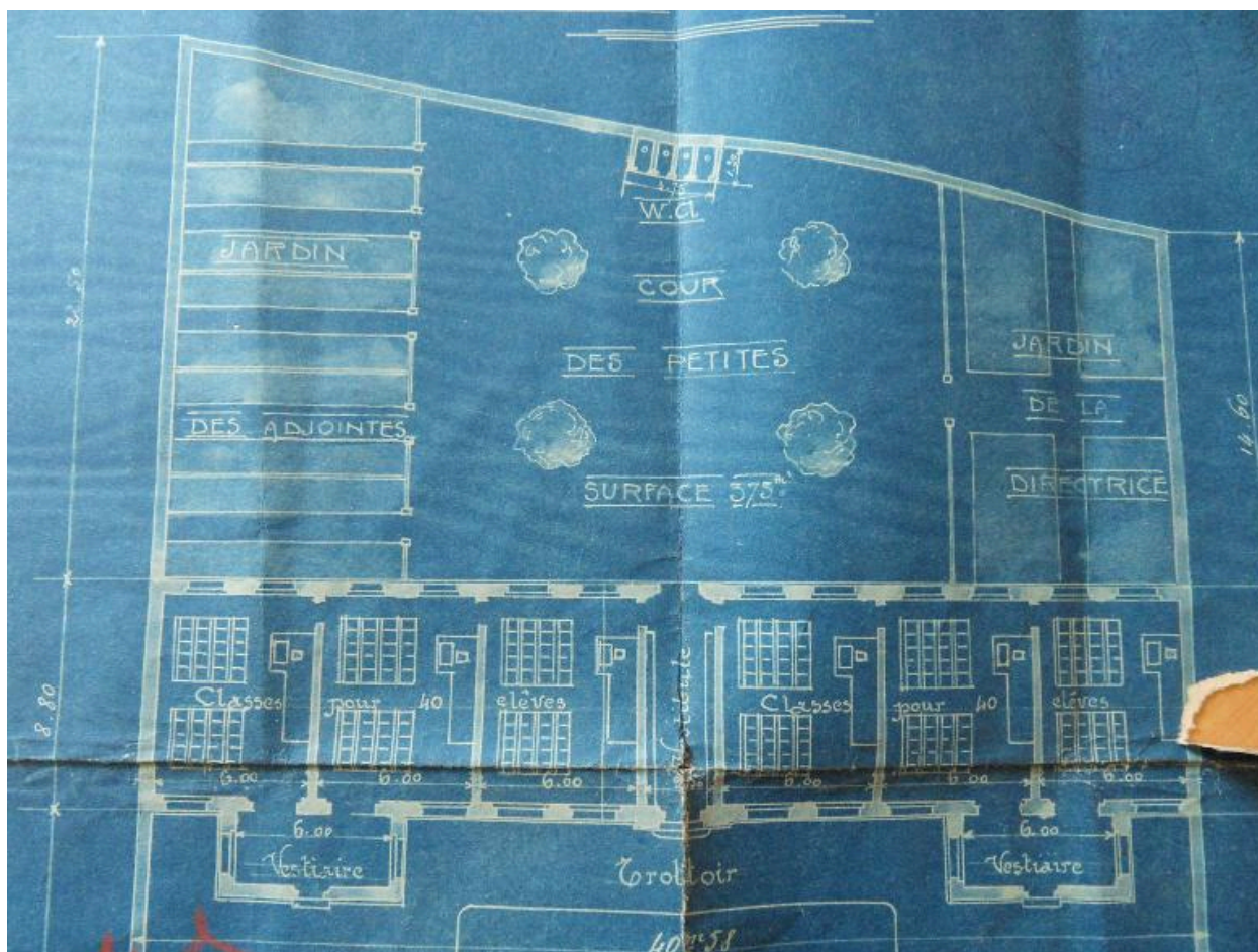
Saint-Ouen. Projet de construction d'une école de filles et de logements pour la directrice et les adjointes. Elévation, plan des salles de classe, Bienaimé architecte, 1906 (AD Somme ; 99O 3405).
