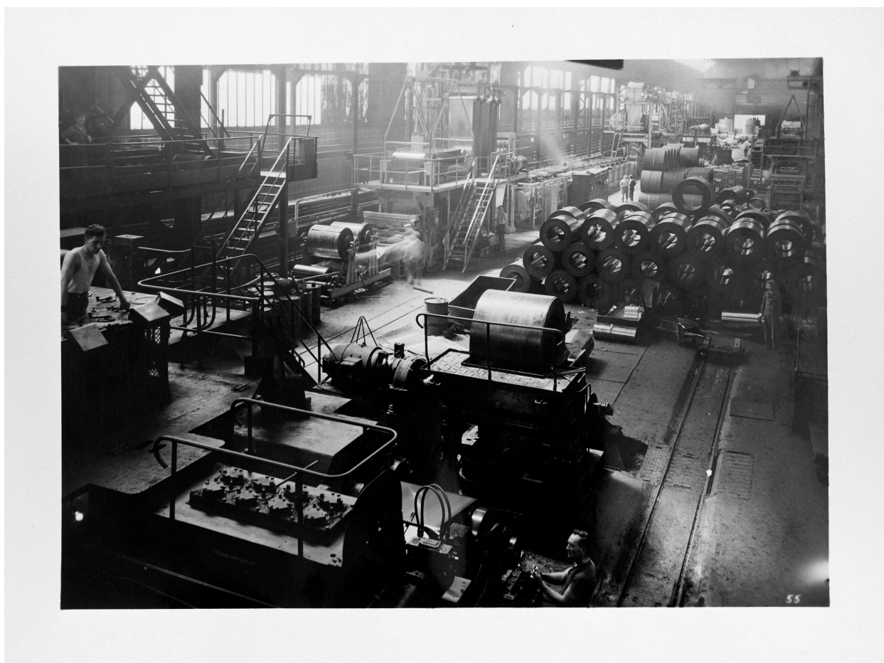
Atelier Rudafer : vue générale du laminoir, trains 1 et 2. Photographie ancienne, auteur inconnu, sans date (coll. part.).
