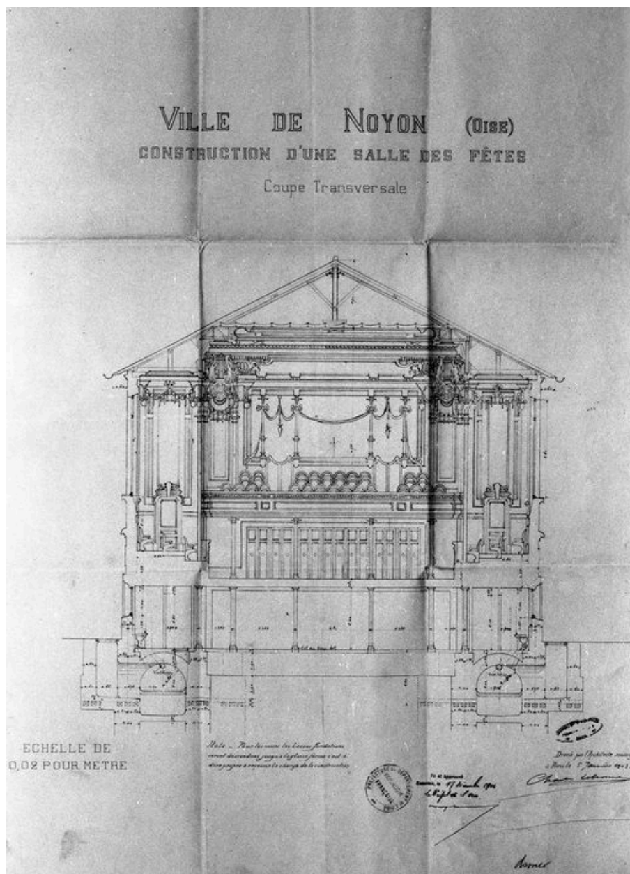
Coupe transversale, projet par C. Lestrone, 1903 (AD Oise ; série O).
