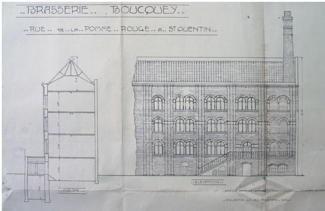
Façade antérieure et coupe transversale des ateliers de fabrication en 1914, par Malgras-Delmas (AD Aisne).
