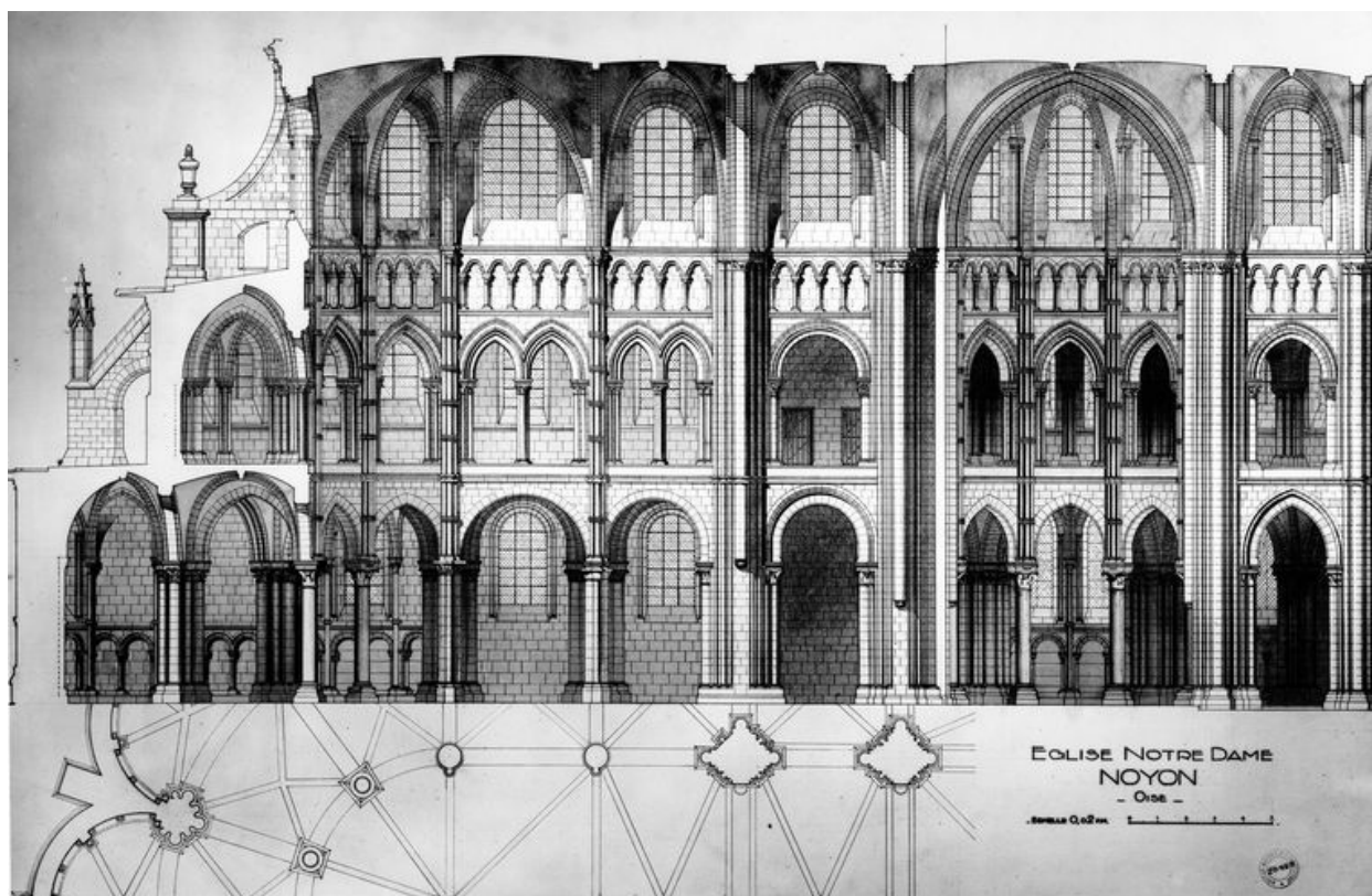
Choeur et transept. Coupe longitudinale et plan partiel, par Collin, 1948.
