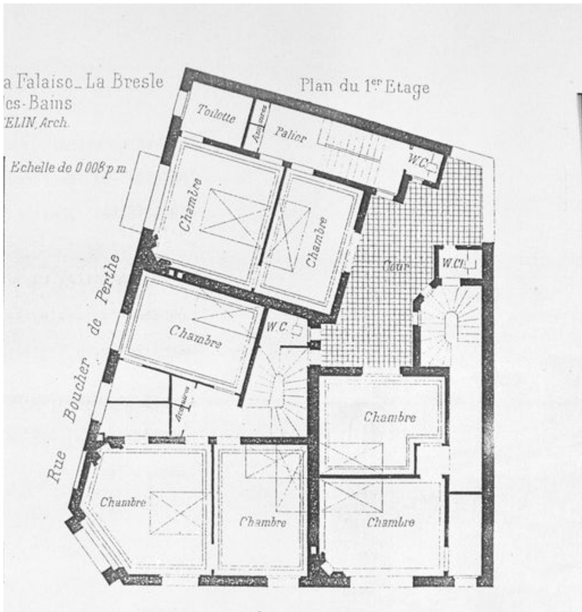
Villas La Prairie, La Falaise, La Bresle, plan du premier étage.
