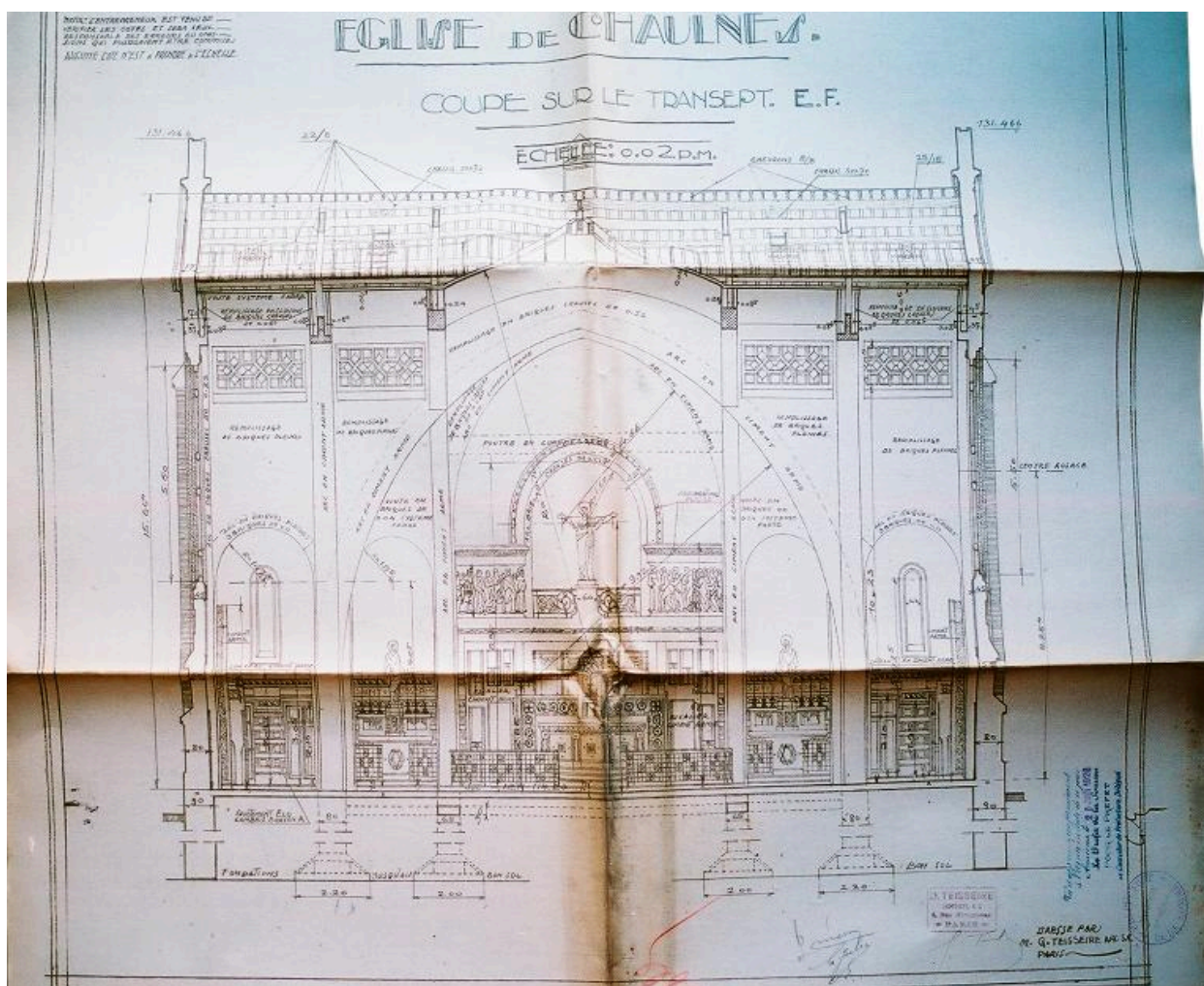
Coupe sur le choeur, 3e projet de reconstruction par Teisseire, 28 juin 1926 (AD Somme ; 99 O 1122).
