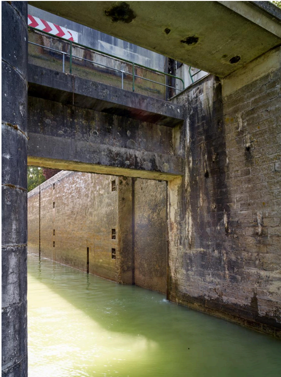
Porte levante en aval et vue du bajoyer maçonné de l'écluse.
