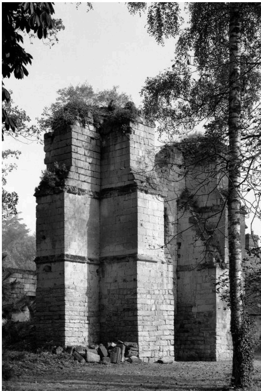
Ouvrage d'entrée. Détail des contreforts.
