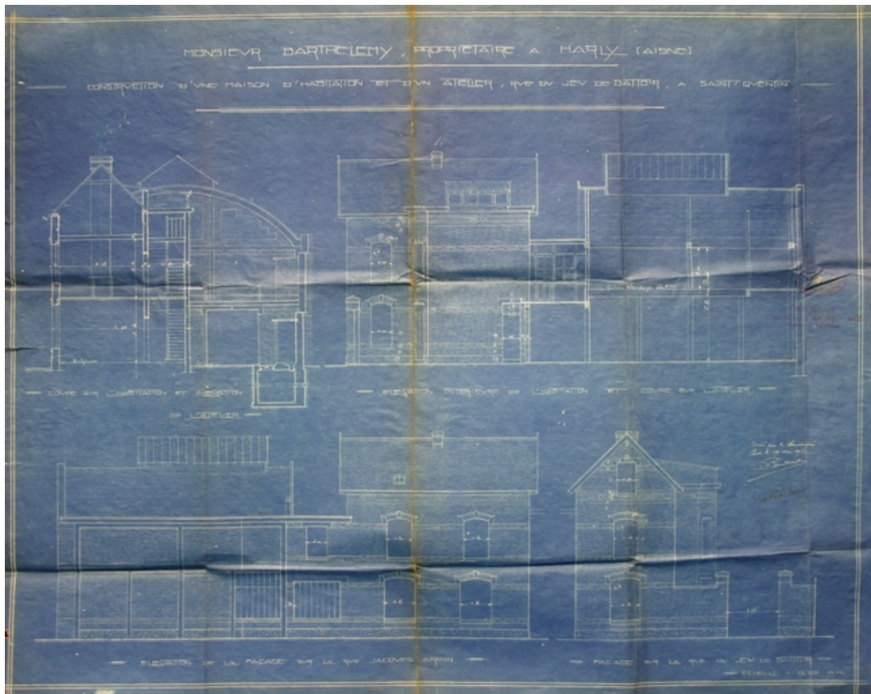
Façades et coupes, par Roulaux, 1922 (AC Saint-Quentin).
