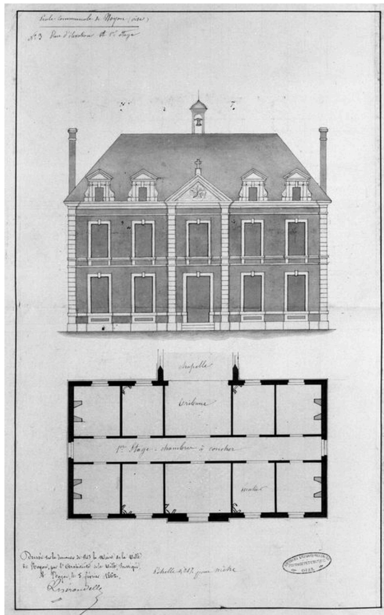
Elévation antérieure et plan du 1er étage, par Lhéronnelle, 1862 (AD Oise ; série O).
