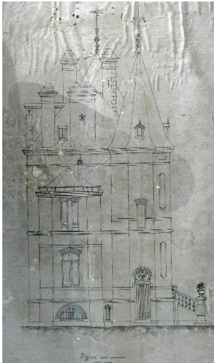
Plan de l'élévation nord-est, dressé par l'architecte Anatole Payen, 1888 (AM Chépy 1M5).
