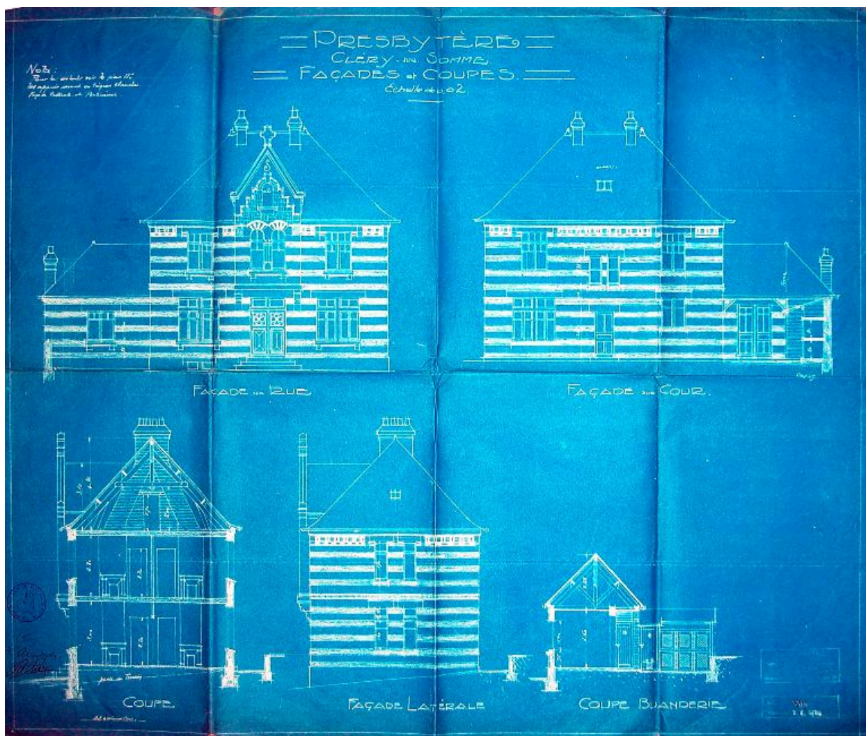
Façades et coupes du presbytère, 3e projet de reconstruction, Emmanuel Chainé (architecte), 1924 (AD Somme ; 99 O 1182).
