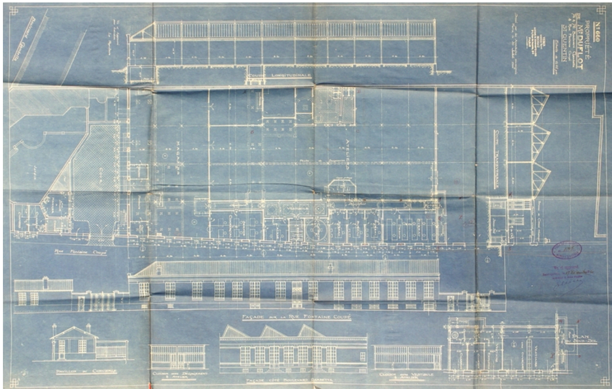
Plans, coupes et élévations des ateliers, par Veber et Michau, 1920 (AC Saint-Quentin).
