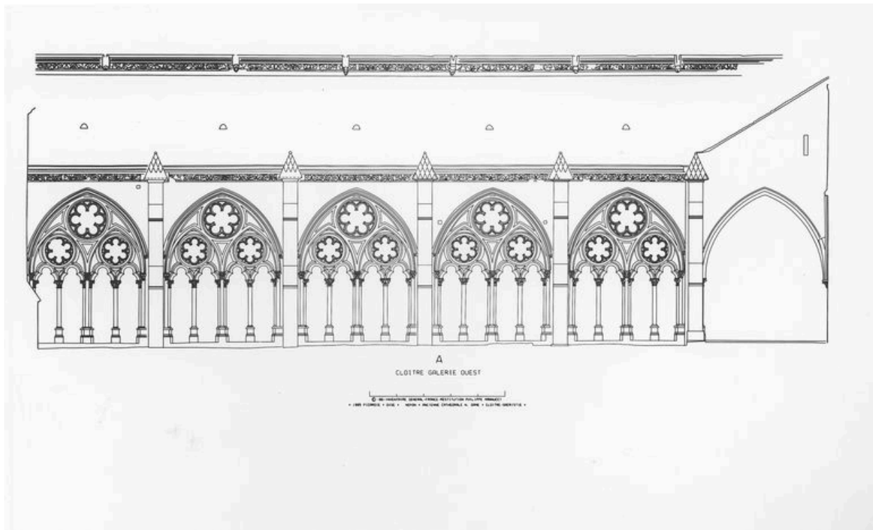
Élévation de la galerie ouest du cloître (relevé photogrammétrique Inventaire général).
