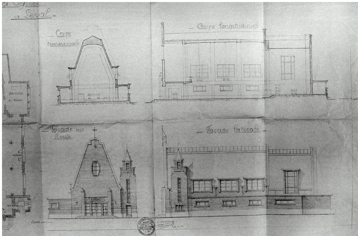
Élévations antérieure et latérale, coupes longitudinale et transversale de la nouvelle église par Fernand Dumont (architecte communal), 25 octobre 1955 (AC Leval ; dossier église).
