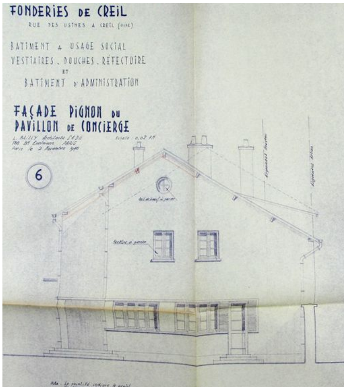
Élévation du mur pignon de la conciergerie, par Bailly, 1946 (AD Oise ; 753W28840).
