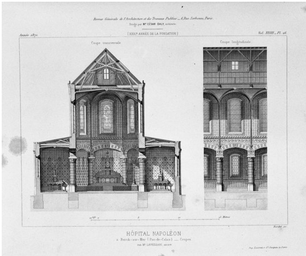
Chapelle, coupe transversale et détail de l'élévation d'une travée du vaisseau central. Rev. gén. de l'arch., t. XXVIII, pl. 26.
