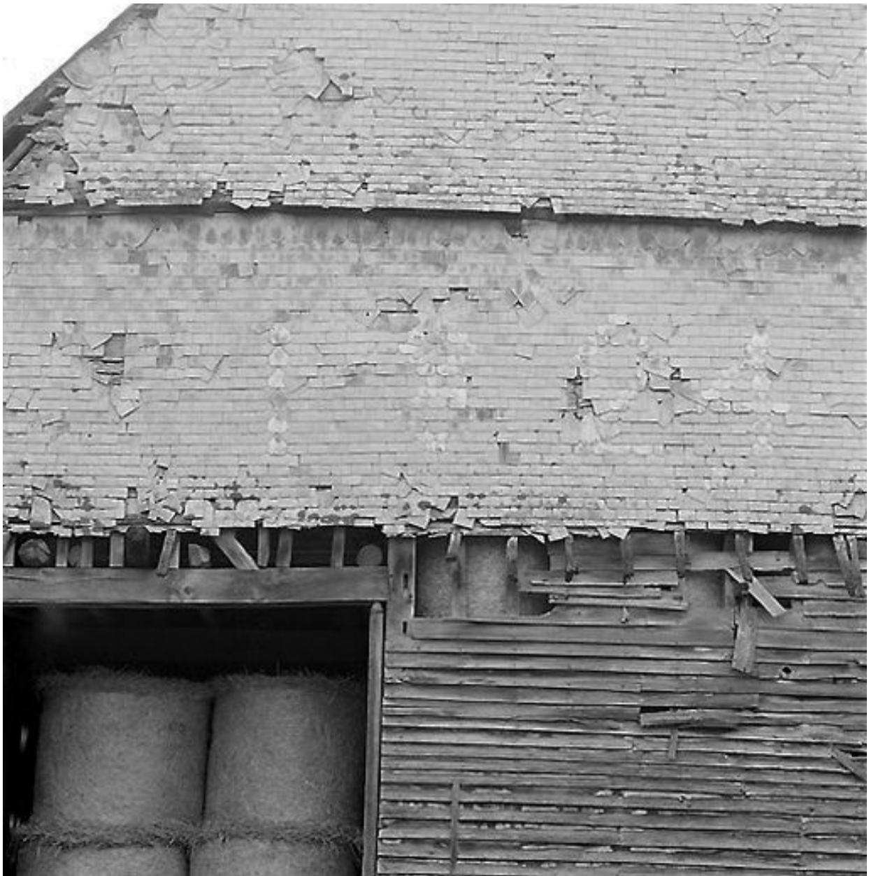
Grange : détail de l'essentage.
